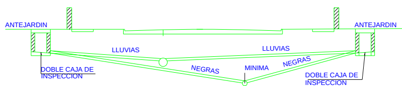
VIA LOCAL - CORTE
