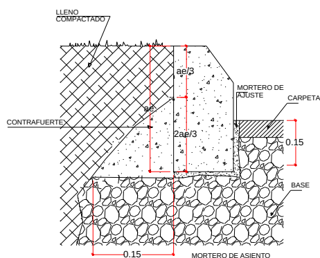
a. bordoillo sobre base del pavimento, respaldo blando.
