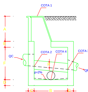
SECCION A-A
