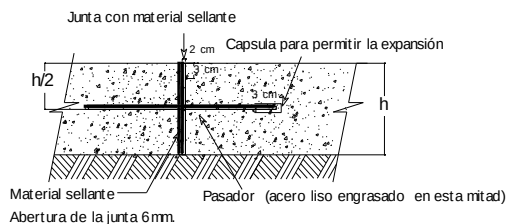
JUNTA DE EXPANSION TIPO 1
