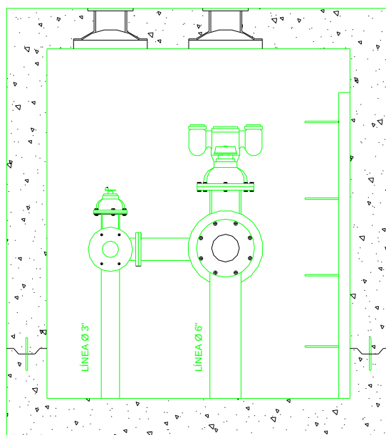
CORTE B-B'
