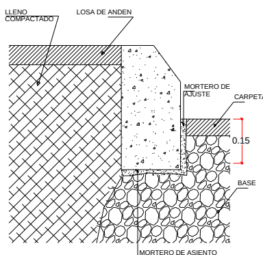
b. bordoillo sobre base del pavimento, respaldo rígido.
