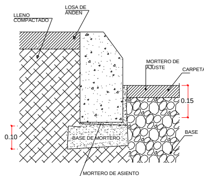
d. bordoillo sobre base de mortero, respaldo rígido.
