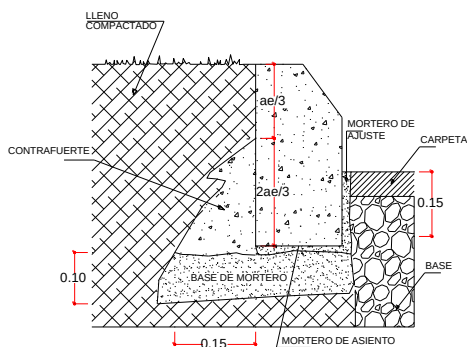
c. bordoillo sobre base de mortero, respaldo blando.
