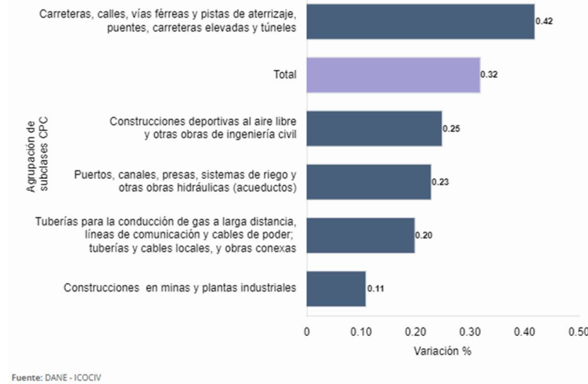
Grafica No. 2 Índice de Costos de la Construcción de Obras Civiles –ICOCIV – mayo 2024
